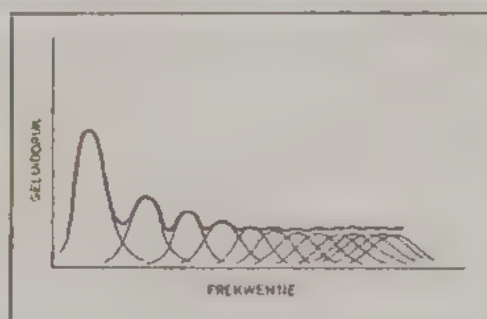
fig. 11 Kamerresponsie en eigentrillingen bij frequentieafhankelijke demping.
